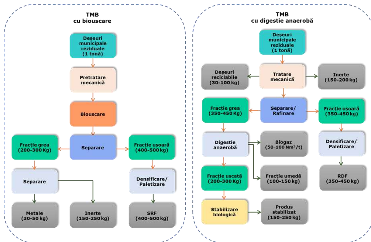
Figura nr. 20 - Fluxul tehnologic al instalațiilor TMB cu biogărare și digestie anaerobă 69
