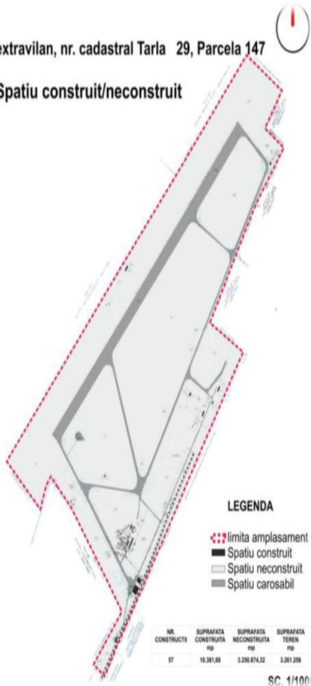
Figura 7 - Tarla 29, parcela 147, nr. cadastral 251, Spațiu construit – neconstruit
