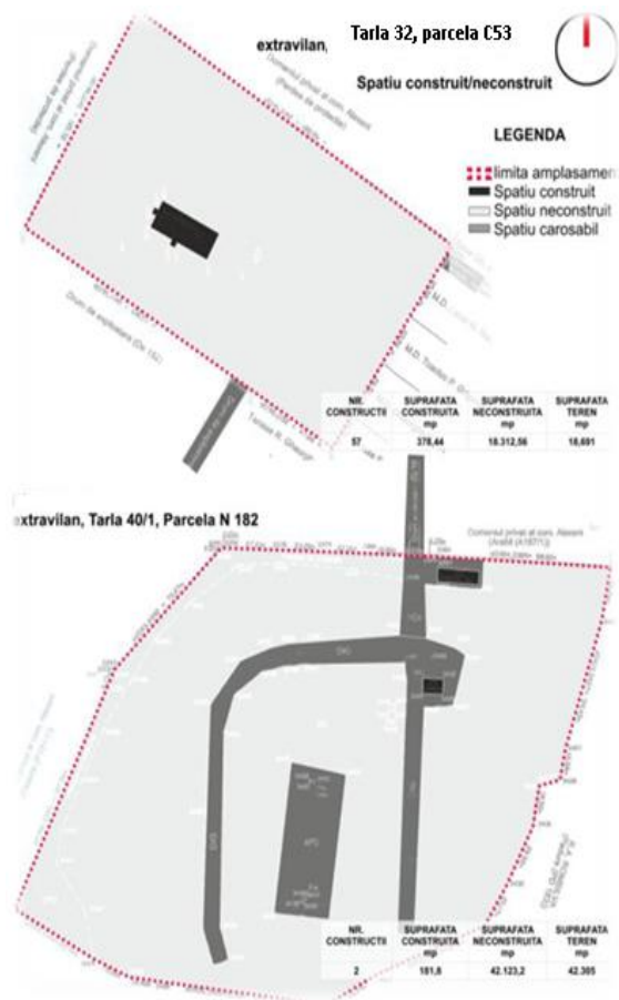
Figura 5 - Tarla 32, parcela C53, nr. cadastral 247, Tarla 40/1, parcela N182, nr. cadastral 248, Spațiu construit – neconstruit
