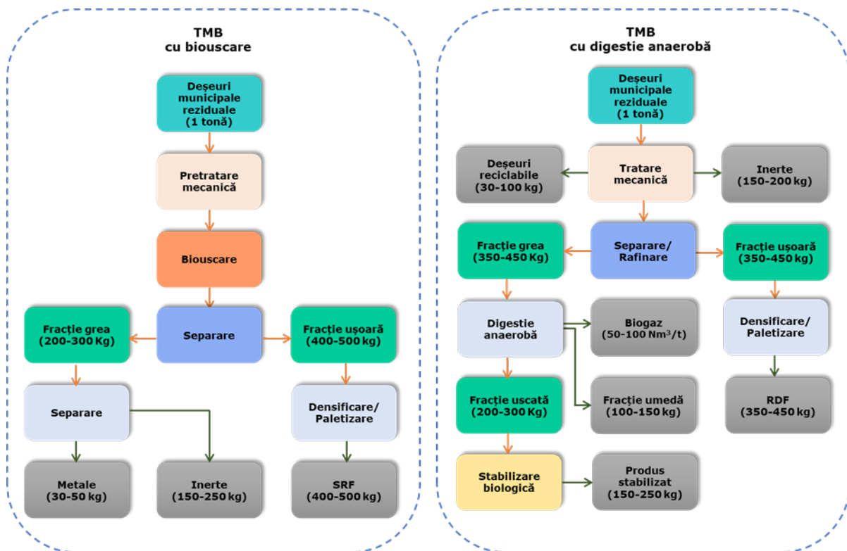
Figura 7-1: Fluxul tehnologic al instalațiilor TMB cu bioușcare și digestie anaerobă 51
